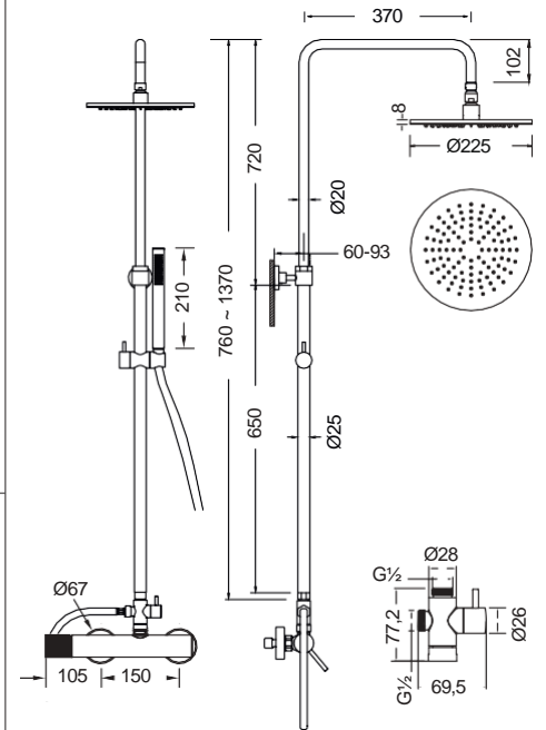
1178066 με κολώνα σταθερού ύψους
